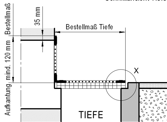
Schnittansicht Tiefe
