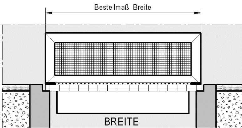
Schnittansicht Breite
